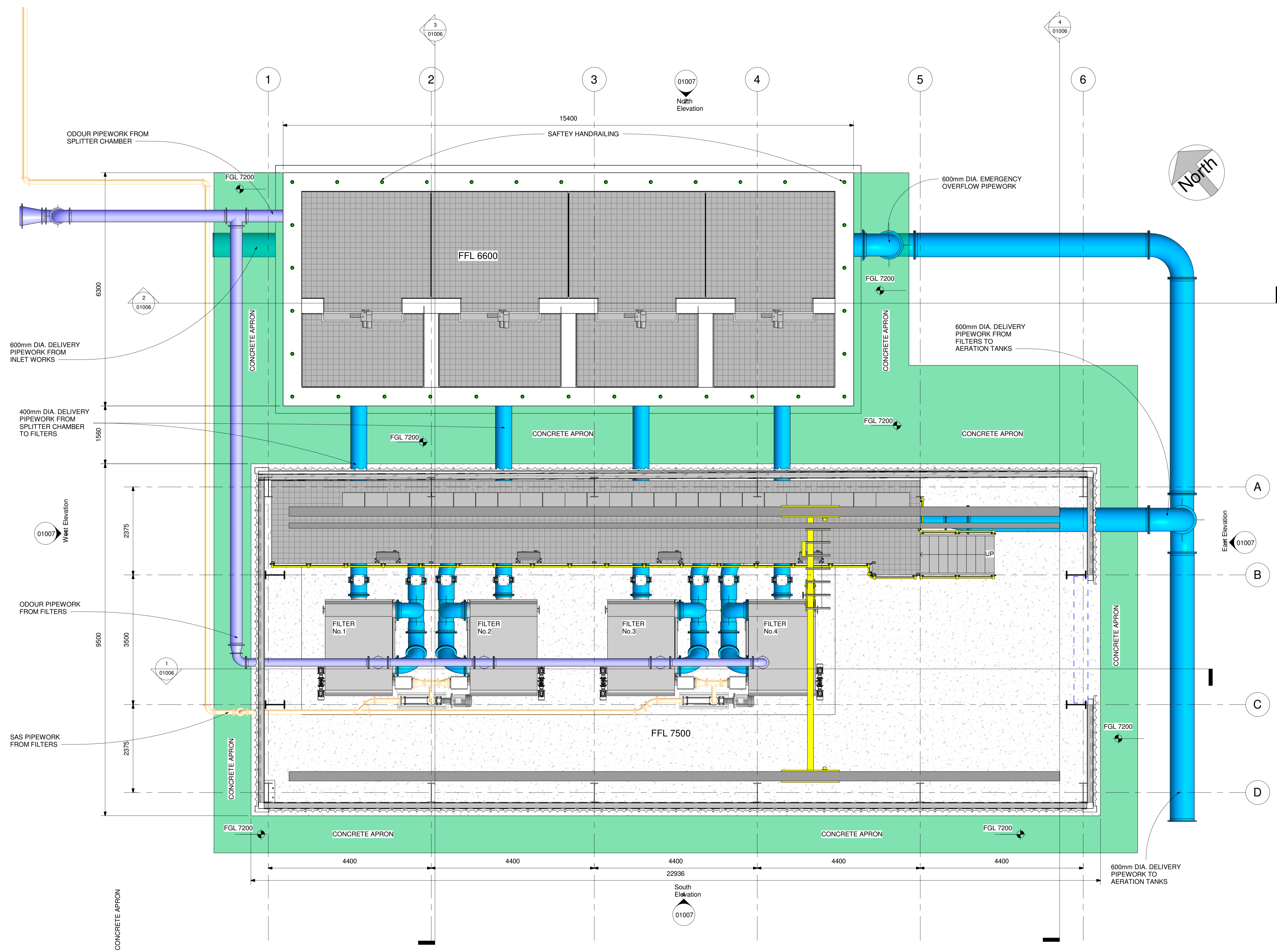
1 FLOOR LAYOUT FFL 1 : 50
